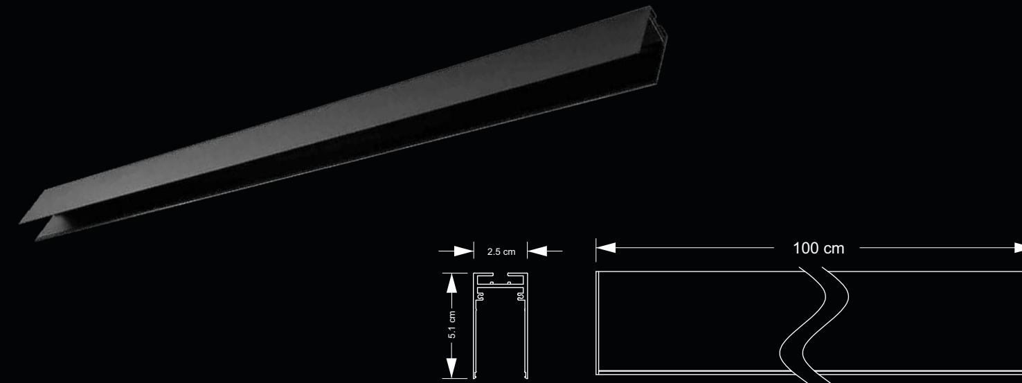
MAGNETIC TRACK ITEM CODE : MG25149 DIMENSION : L 100 cm X W 2.5 cm X H 5.1 cm
